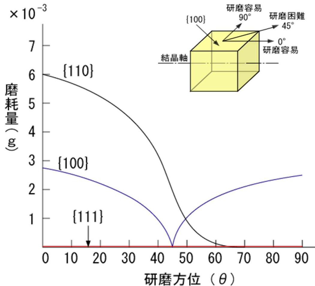
【摩耗曲線】
